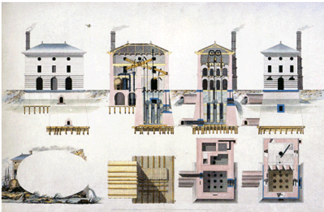
afb. 19. Jan Blanken, 'Stoommachine- en pompgebouw te Hellevoetsluis', ca. 1799-1800.
