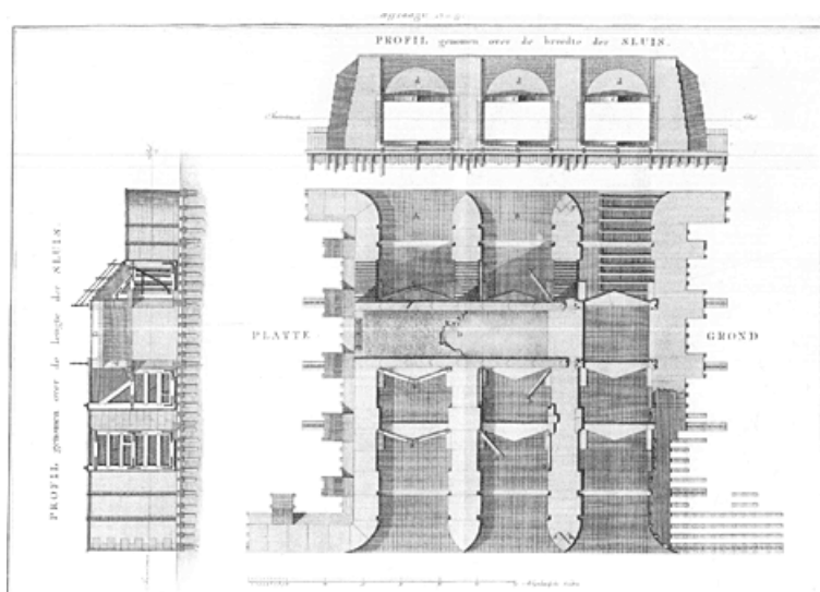
afb. 9. D. Veelwaard, 'Profil genomen over de lengte der sluis / Profil genomen over de breedte der sluis' [bij Katwijk aan zee].
